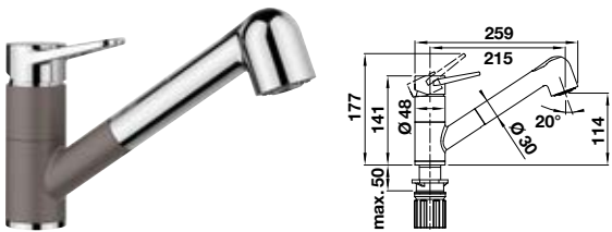
Auslauf 180° schwenkbar mit Schlauchbrause, umstellbar
