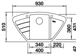
Ausschnitt nach Schablone Beckentiefe: 180 mm Außenmaß: 930 x 510 mm
