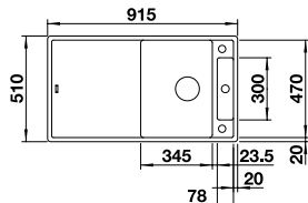
Ausschnitt: 895 x 490 mm Beckentiefe: 190 mm Außenmaß: 915 x 510 mm
