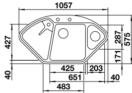
Ausschnitt nach Schablone Beckentiefe: 185/120 mm Außenmaß: 575 x 1057 mm
