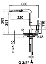
Kaltstart Auslauf 140° schwenkbar mit umstellbaren Schlauchauszug
