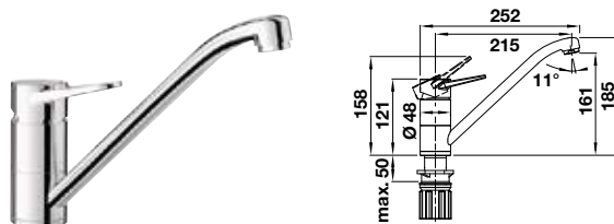
Auslauf 180° schwenkbar
