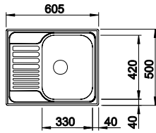
Ausschnitt: 587 x 482 mm Beckentiefe: 160 mm Außenmaß: 605 x 500 mm
