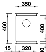
Ausschnitt: 320 x 400 mm Beckentiefe: 190 mm Außenmaß: 350 x 460 mm
