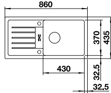
Ausschnitt: 840 x 415 mm Beckentiefe: 180 mm Außenmaß: 860 x 435 mm
