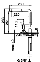
Kaltstart Auslauf 140° schwenkbar mit Schlauchauszug, Metallschlauch, Hebel links
