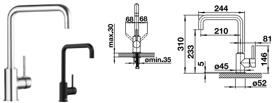
Auslauf 360° schwenkbar
