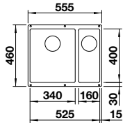
Ausschnitt: 525 x 400 mm Beckentiefe: 190/130 mm Außenmaß: 555 x 460 mm
