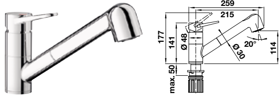
Auslauf 180° schwenkbar mit Schlauchbrause, umstellbar
