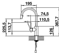
Kaltstart Auslauf 190° schwenkbar mit Schlauchauszug
