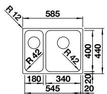
Ausschnitt: 545 x 400 mm Beckentiefe: 130/185 mm Außenmaß: 585 x 440 mm
