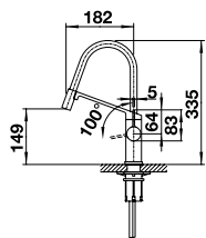
Kaltstart Auslauf 360° schwenkbar mit beweglichem Schlauch
