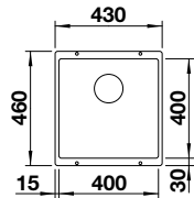
Ausschnitt: 400 x 400 mm Beckentiefe: 190 mm Außenmaß: 430 x 460 mm
