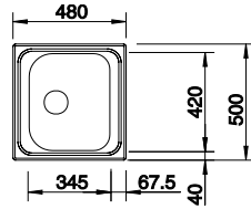
Ausschnitt: 462 x 482 mm Beckentiefe: 160 mm Außenmaß: 480 x 500 mm
