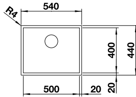
Ausschnitt: 500 x 400 mm Beckentiefe: 175 mm Außenmaß: 540 x 440 mm
