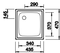
Ausschnitt: 417 x 452 mm Beckentiefe 150 mm Außenmaß 435 x 470 mm
