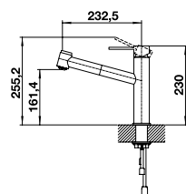
Auslauf 130° schwenkbar mit umstellbaren Schlauchauszug
