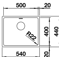
Ausschnitt: 500 x 400 mm Beckentiefe: 190 mm Außenmaß: 540 x 440 mm
