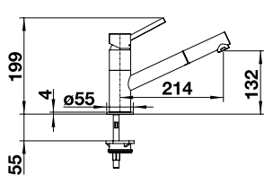
Kaltstart Auslauf 120° schwenkbar mit Schlauchauszug
