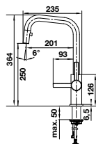
Kaltstart Auslauf 190° schwenkbar mit Schlauchauszug
