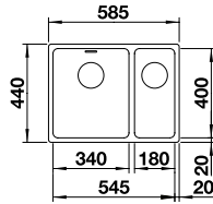
Ausschnitt: 545 x 400 mm Beckentiefe: 190 mm Außenmaß: 585 x 440 mm
