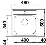
Ausschnitt: 462 x 482 mm Beckentiefe: 158 mm Außenmaß: 480 x 500 mm
