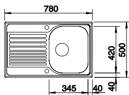
Ausschnitt: 762 x 482 mm Beckentiefe: 160 mm Außenmaß: 780 x 500 mm
