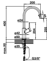
Kaltstart Auslauf 190° schwenkbar mit Schlauchauszug
